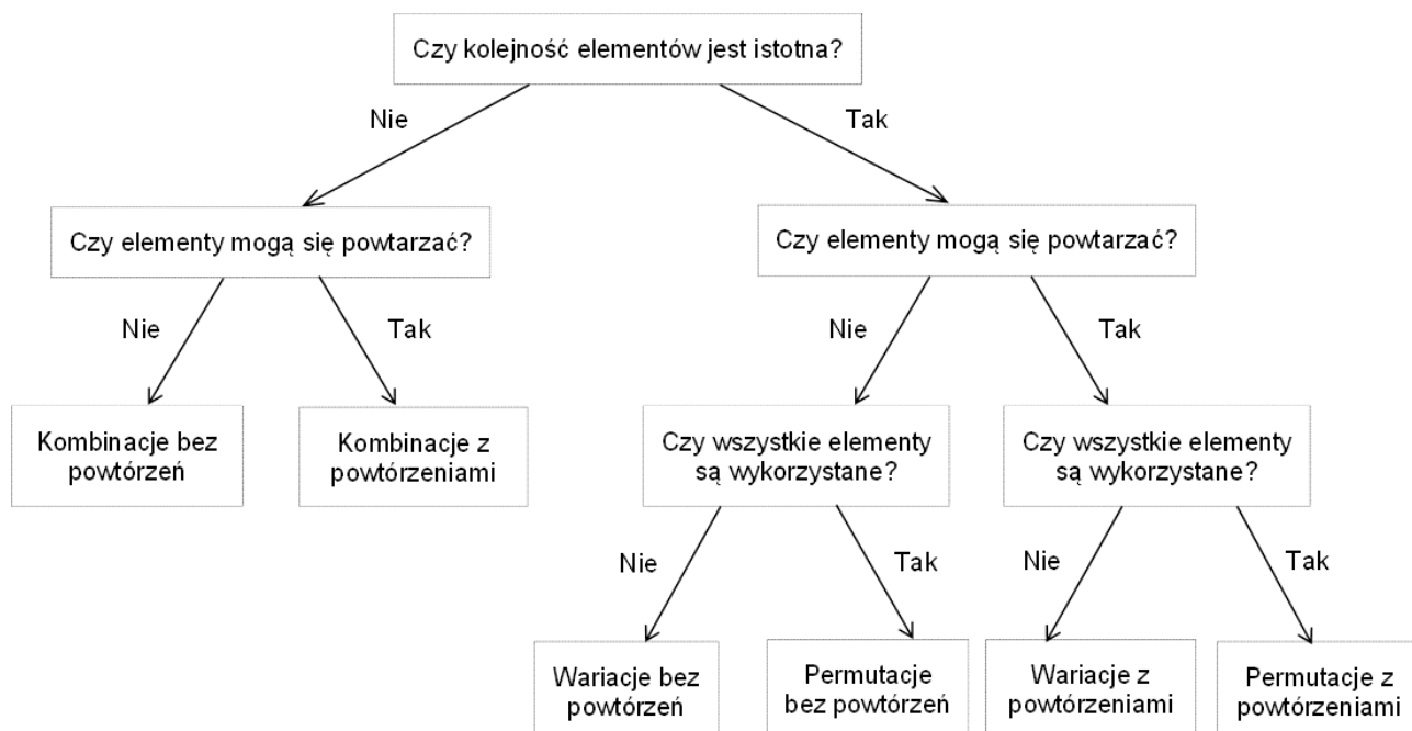
Rys. 1. Podstawowy schemat postępowania w kombinatoryce.
