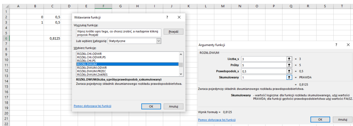
Rys.10. Obliczanie prawdopodobieństwa z rozkładu dwumianowego za pomocą funkcji ROZKŁ.DWUM( ; ; ; )
