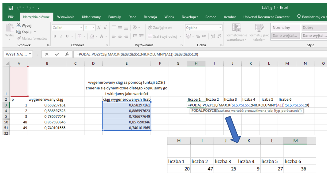
Rys. 6. Wynik omawianego schematu
